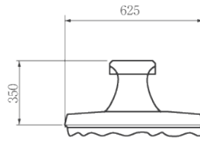
天端型 1/4
