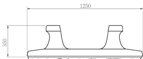
天端型
